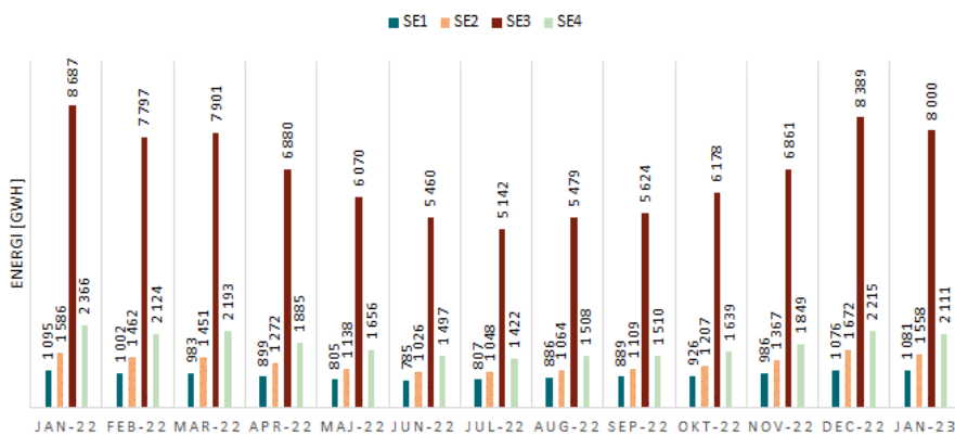
Figur 5 Elanvändning per elområde och månad för 2022 och januari 2023
