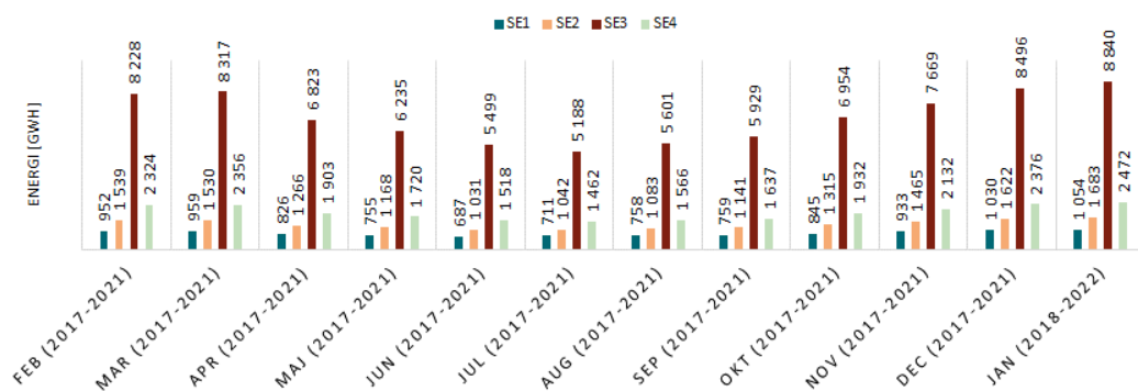
Figur 4 Genomsnittlig faktisk elanvändning för referensperioden per elområde och månad för åren
