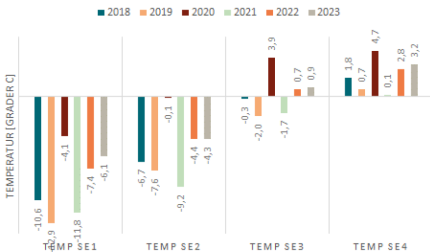
Figur 8 Viktad temperatur för elområden i januari
