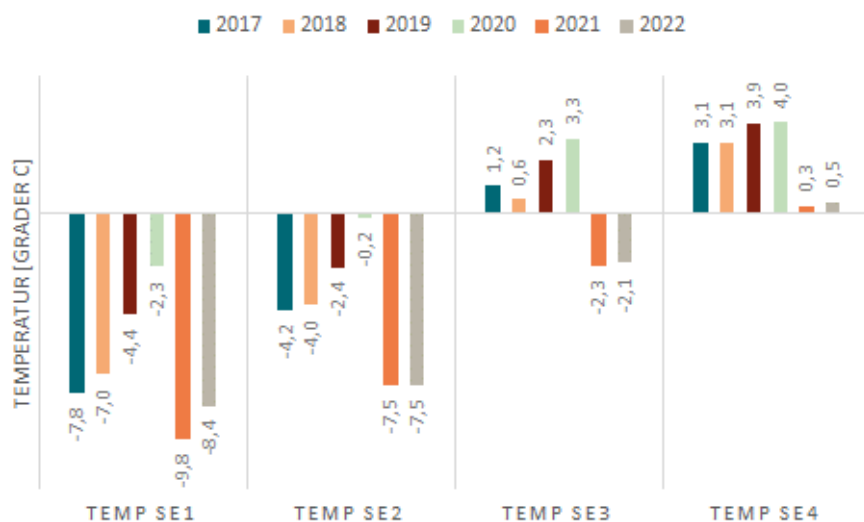
Figur 9 Viktad temperatur för elområden i december
