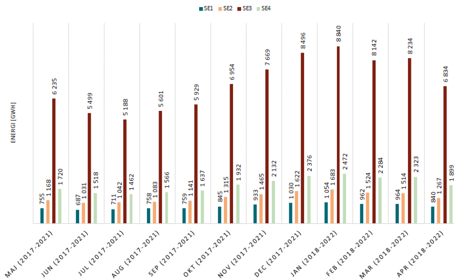
Figur 4 Genomsnittlig faktisk elanvändning för referensperioden per elområde och månad
