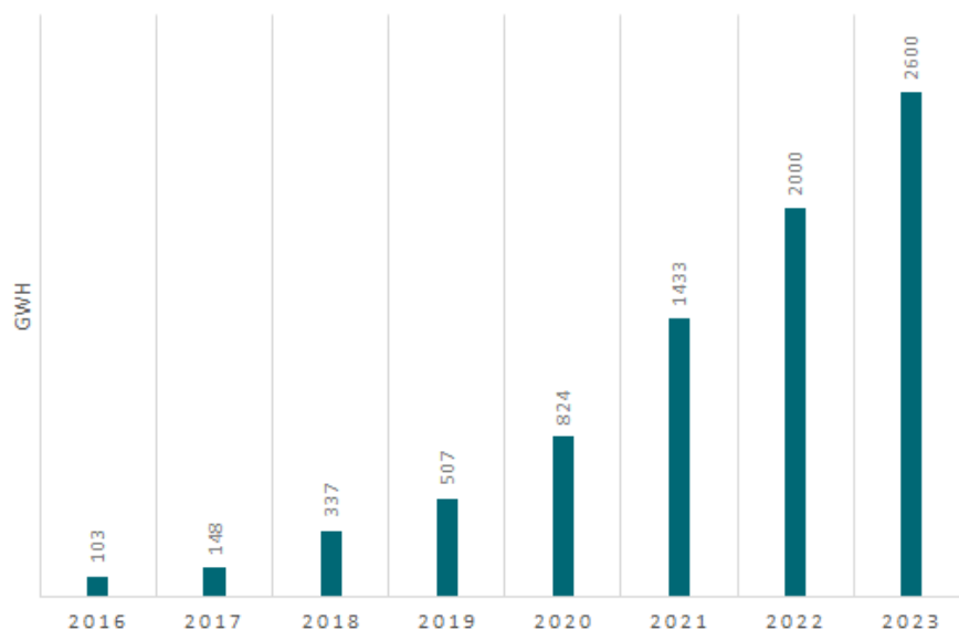
Figur 22 Elanvändning till vägtrafik per år, statistik 2016–2021, prognos 2022–2023
