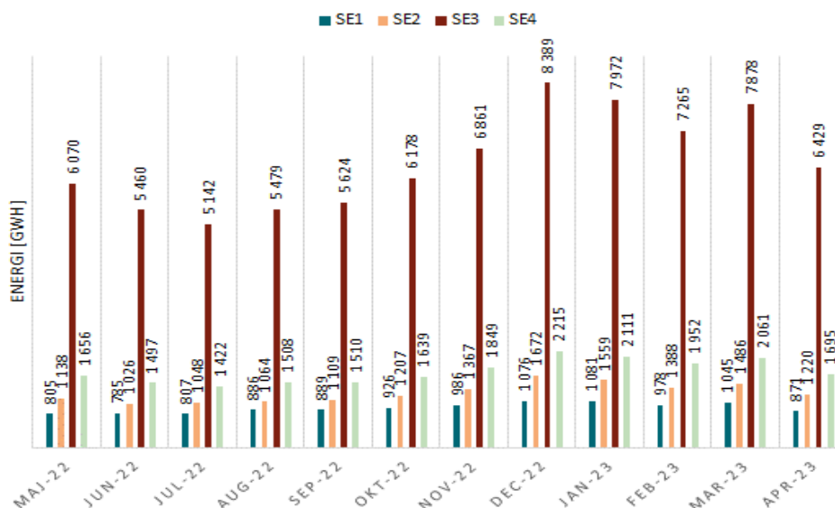
Figur 5 Faktisk elanvändning per elområde och månad
