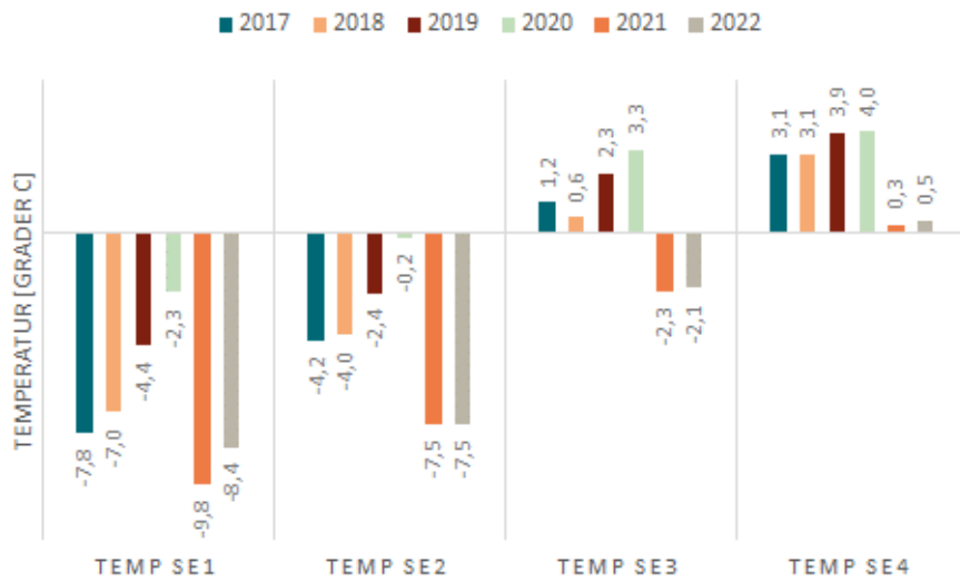
Figur 12 Viktad temperatur för elområden i december
