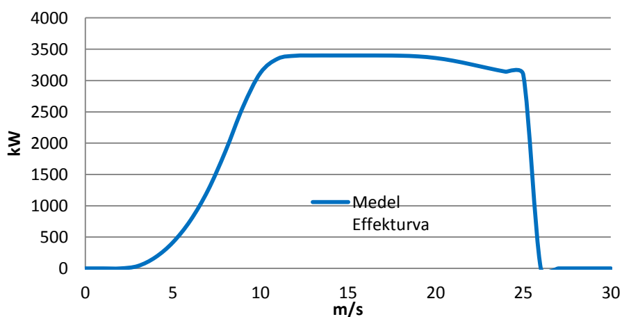
Figur 3.3 Genomsnittlig effektkurva som använts i potentialberäkningarna. Källa: egen bearbetning av data från Siemens, Vestas och Gamesa.
