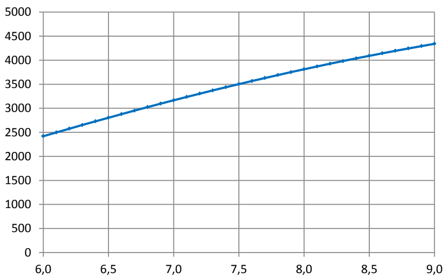
Figur 3.4 visar hur antalet fullasttimmar varierar med medelvindhastigheten. Kurvan är netto och beräknad utifrån referenseffektkurvan och ett anslag om 14 % förluster.
