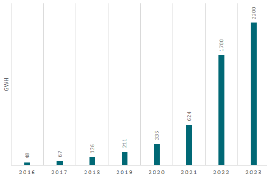
Figur 25 Elanvändning till vägtrafik per år, statistik 2016–2021, prognos 2022–2023
