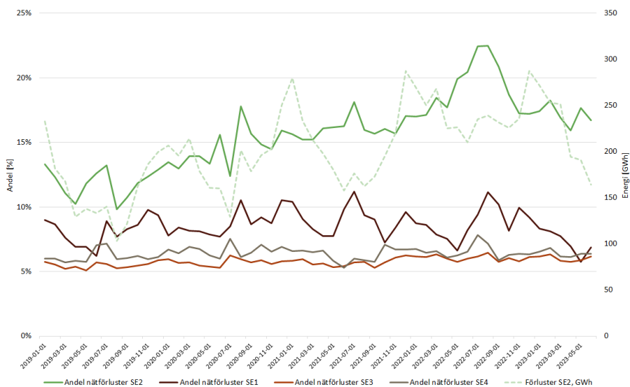
Figur 24 Utveckling av andelen nätförluster, procent och GWh t.o.m juni 2023
