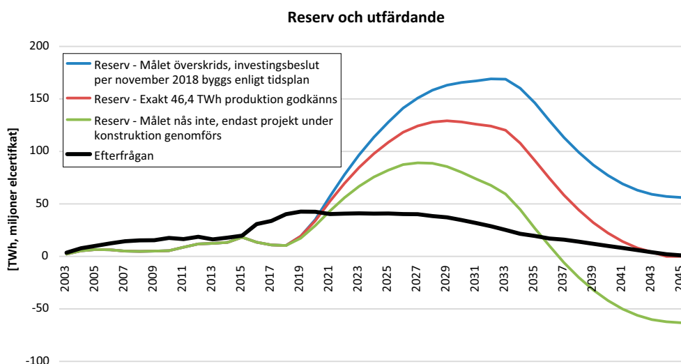
Figur 2. Exempel på reservens utveckling samt tilldelning av elcertifikat i Sverige och Norge fram till 2045 för olika utbyggnadsscenarioer. Scenariot där det byggs mer än 46,4 TWh avser projekt med investeringsbeslut i Norge och Sverige som inte ännu har påbörjat byggnation.
