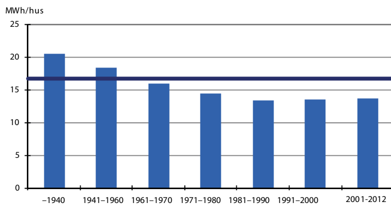
Figur 2 Genomsnittlig energianvändning per småhus (för uppvärmning och varmvatten, exkl. hushållsel) under år 2013, fördelad efter husets byggår, MWh/hus
