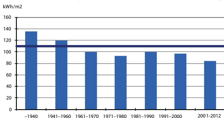
Figur 3 Genomsnittlig energianvändning per kvadratmeter (för uppvärmning och varmvatten, exkl. hushållsel) i småhus under år 2013, fördelad efter byggår, kWh/m 2
