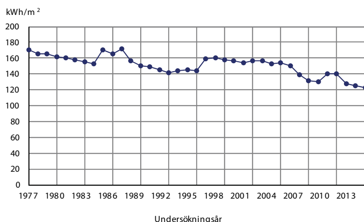
Figur 4 Genomsnittlig elanvändning (inkl. hushållsel) i småhus uppvärmda enbart med el, år 1977-2013, kWh/m 2
