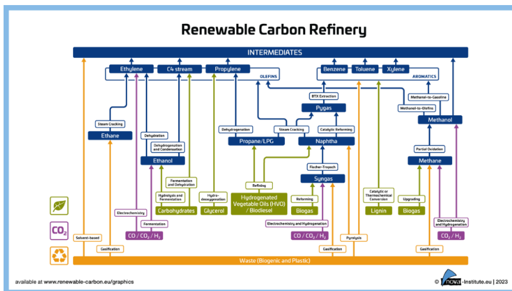
Figur 5. Produktionsvägar och råvaror för tillverkning av eten och propen, Nova-institut 10
