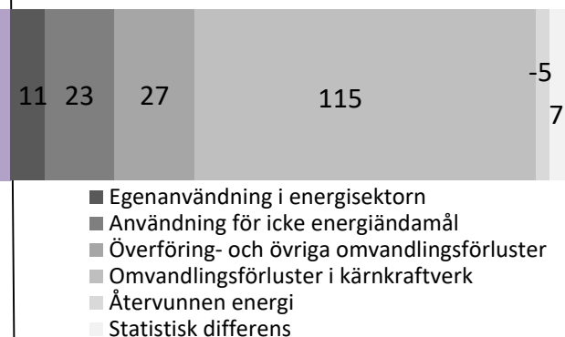
Förluster, annan användning och statistisk differens, 179 TWh
