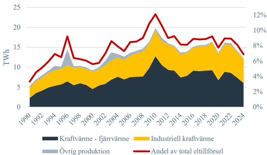
Figur 1. Bruttotillförsel av elenergi i TWh per år efter produktionsslag, vänster axel. Inom kategorin Övrigt ingår kondens- samt gasturbinproduktion. Linjen visar andel av total bruttotillförsel av elenergi som utgörs av konventionell kraftvärme, höger axel. Under perioden 1990–2024.
