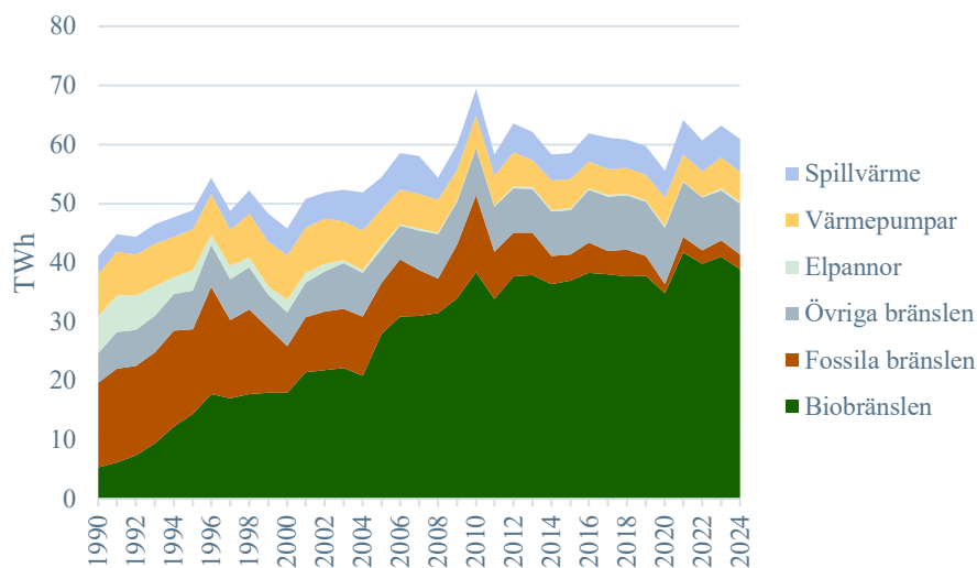
Figur 2. Tillförd energi för fjärrvärmeproduktion per kategori i TWh per år under perioden 1990–2024. I kategorin Fossila bränslen ingår petroleumprodukter, naturgas samt kol inkl. koks- och masugns gas.
